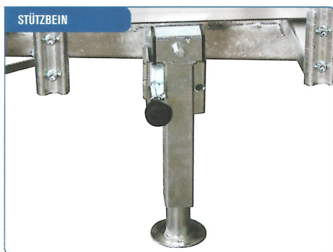
STÜTZBEIN Die kräftige Klappkurbelstütze, sorgt für sicheres und stabiles be- und entladen. 2 Stück als Set, inkl. Handkurbel.
